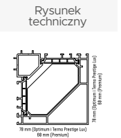
Przekrój łącznika kątownego Termo 90°
