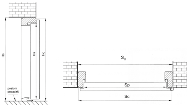
Sposób wymiarowania drzwi z ościeżnicą "11", "12" oraz TERMO i TERMO PRESTIGE
