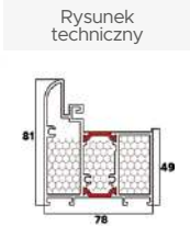
Ościeżnica "9" Premium / Normal
