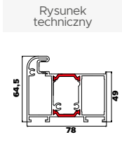
Ościeżnica "11" Premium / Normal
