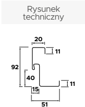
Ościeżnica "9" Premium / Normal
