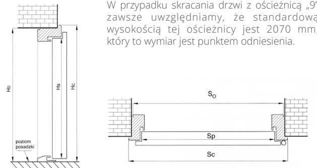
Sposób wymiarowania drzwi z ościeżnicą "9"
