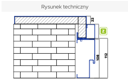
Złożenie ościeżnicy "11" Protect z łącznikiem portalu
