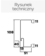
Ościeżnica "11" Premium / Normal
